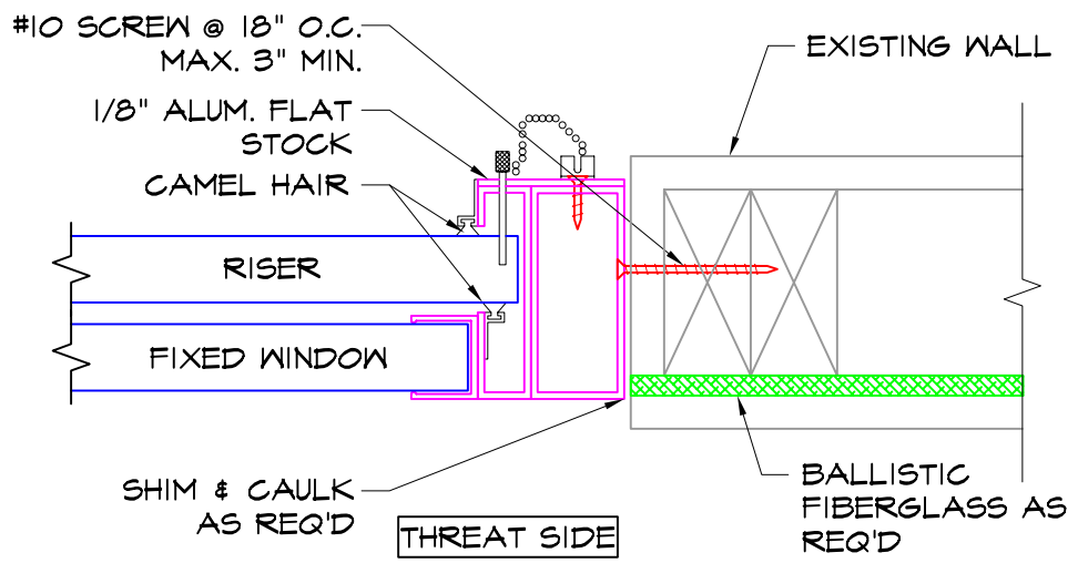
# WINDOW JAMB RISER 3"=1'-0"
